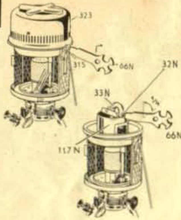
Bild 5 Regulieren der Heizflamme und Einstellen der Lichtstärke
