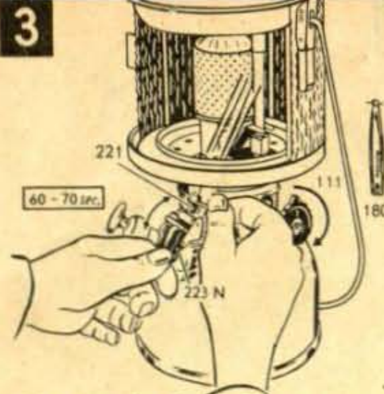
Bild 3 Anzünden des Gerätes
