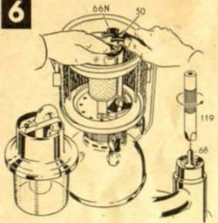
Bild 6 Auswechseln der Düse (50) bzw. Reinigungsnadel (68)
