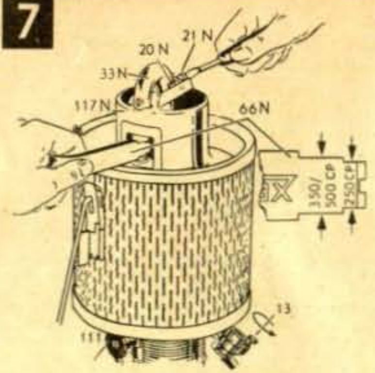
Bild 7 Einstellen des richtigen Mischrohrabstandes
